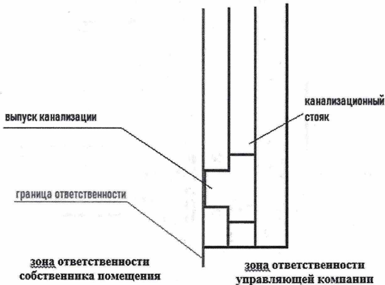
Схема №3. Система водоотведения хозяйственно-бытовых отходов
