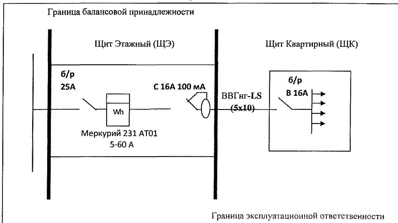
Электрическая схема
