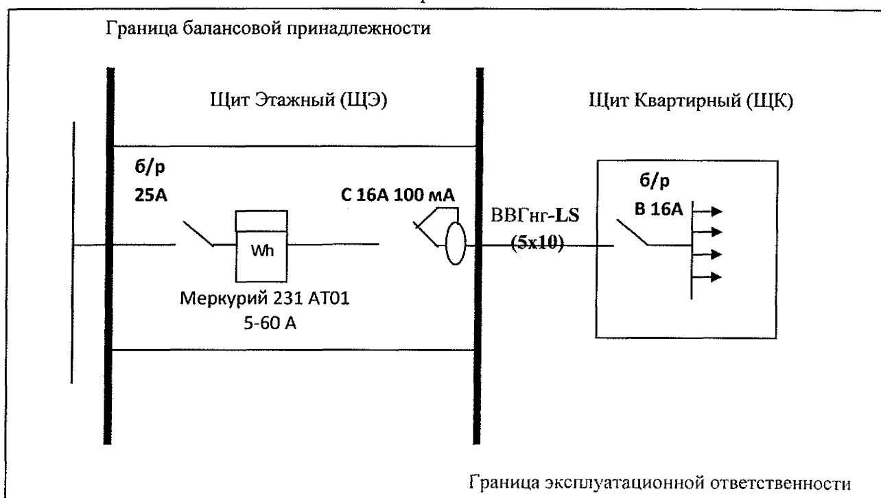
Электрическая схема
