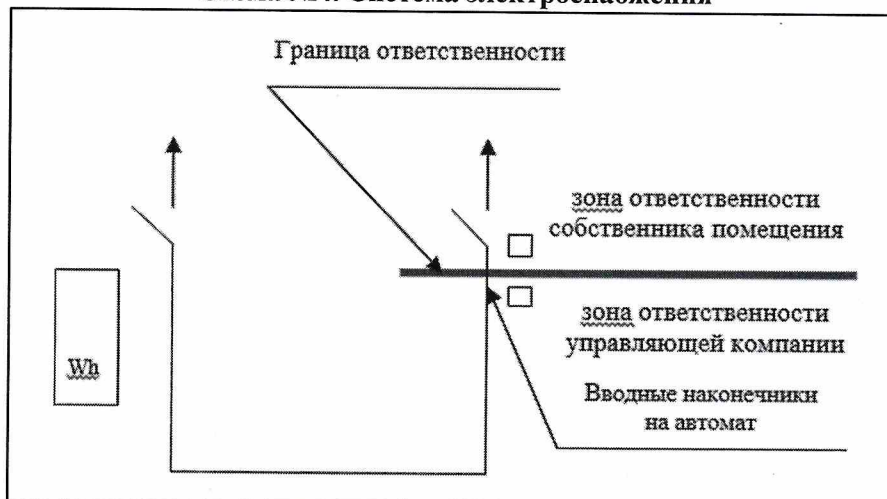
Схема №4. Система электроснабжения
