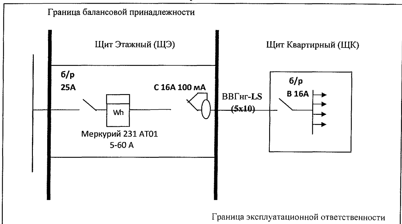
Электрическая схема
