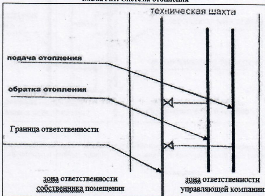
Схема №1. Система отопления
