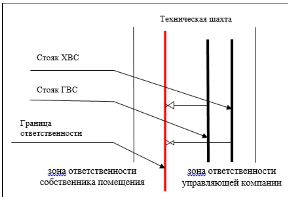
Схема №2. Системы холодного и горячего водоснабжения
