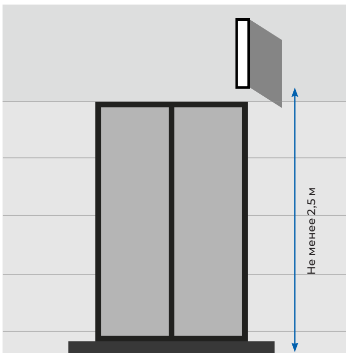
Панель-кронштейн (вид сбоку)
