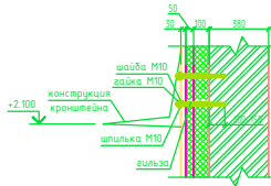
Крепление конструкции кронштейна для наружного кондиционера
