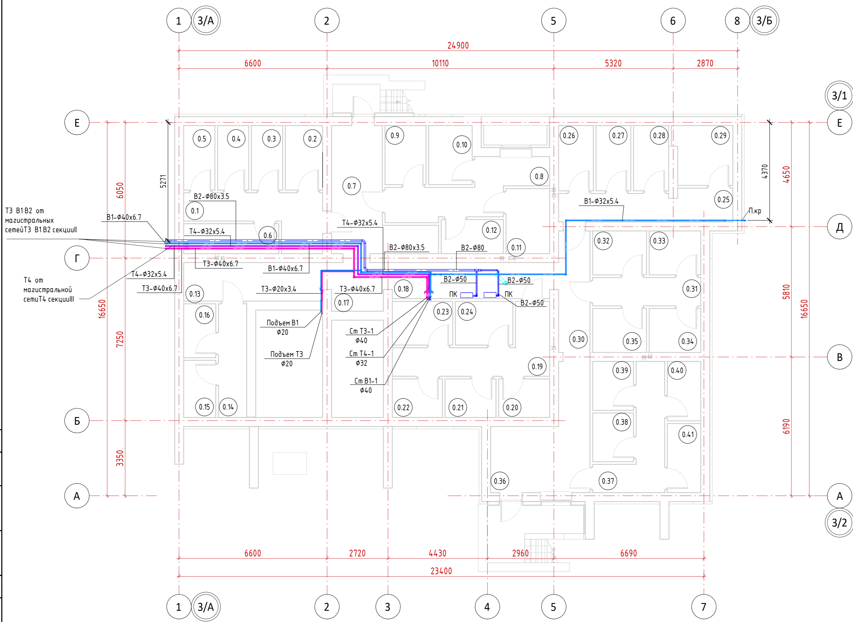
Схема расположения секций
