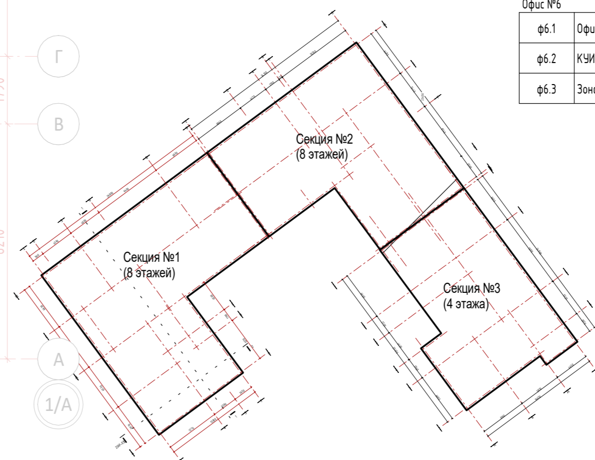
Схема расположения секций
