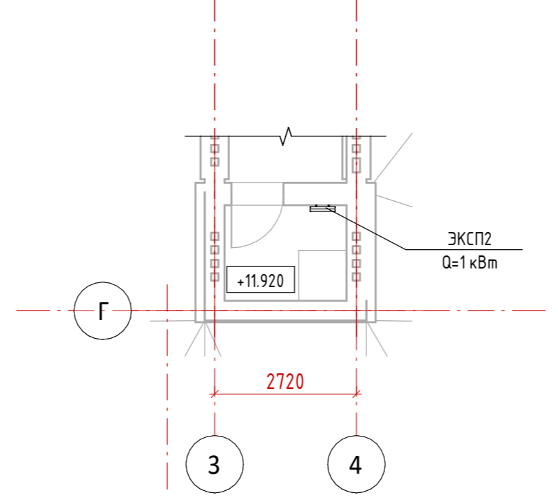
Фрагмент плана кровли на отм. 11.920
