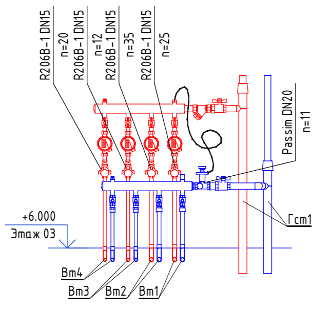
Настройки регулирующей арматуры УЧ1.3
