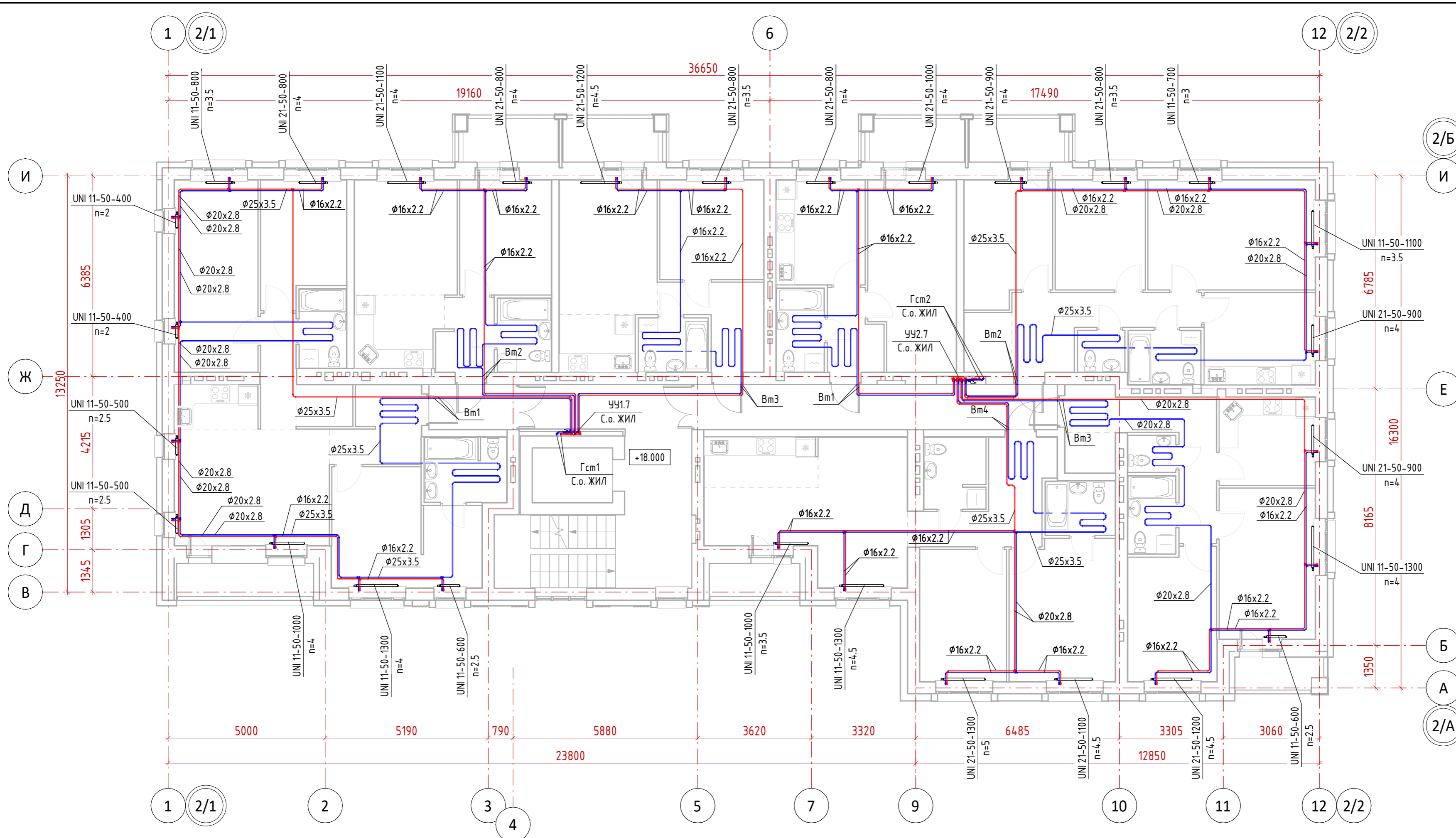
Настройки регуливающей арматуры УЧ1.7
