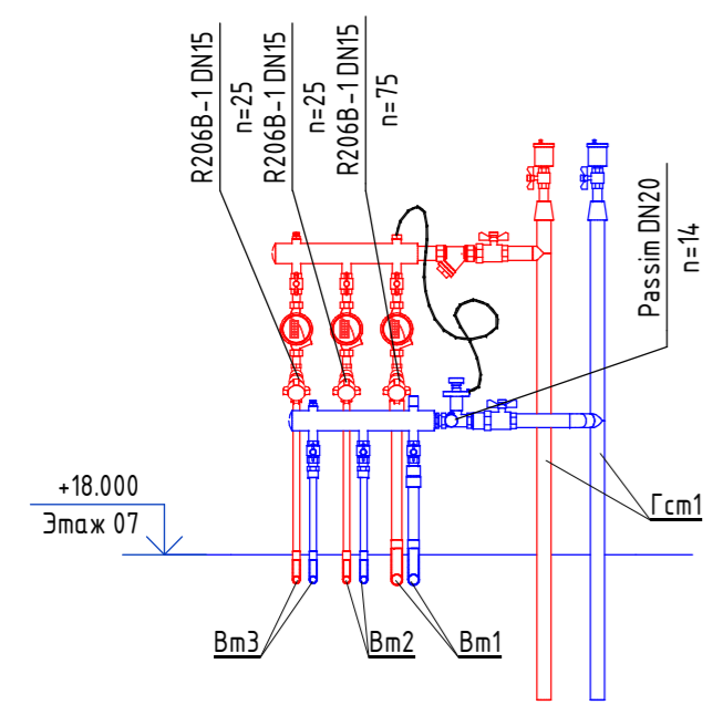
Настройки регуливающей арматуры УЧ1.7
