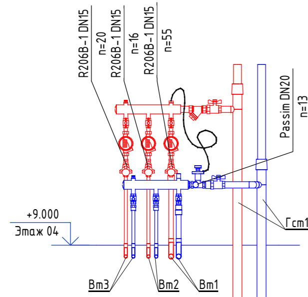
Настройки регулирующей арматуры УЧ1.4
