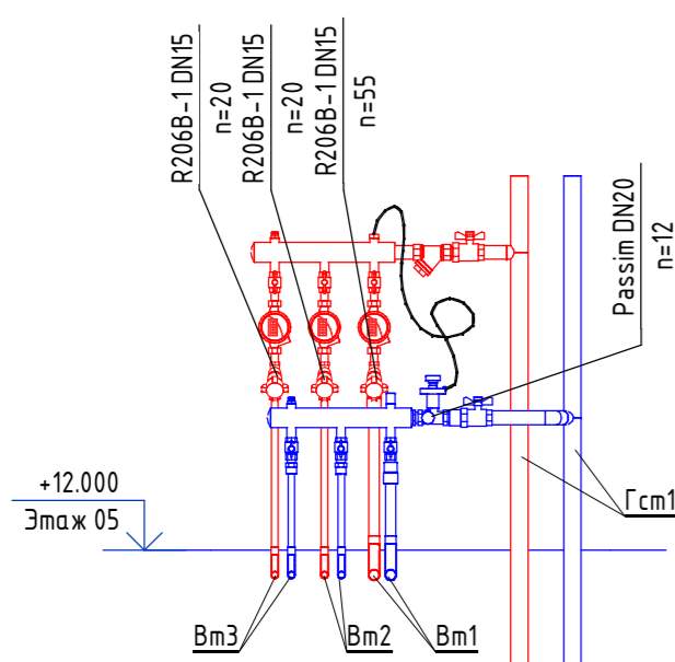
Настройки регулирующей арматуры ЧУ1.5
