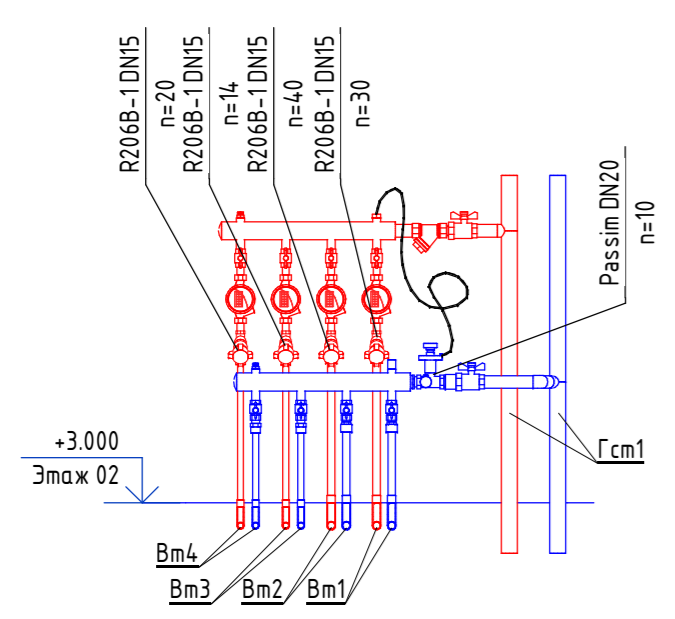
Настройки регулирующей арматуры УЧ1.2
