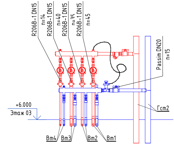
Настройки регулирующей арматуры УЧ2.3
