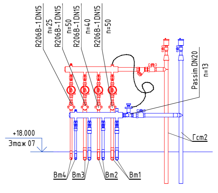
Настройки регуливающей арматуры УЧ2.7
