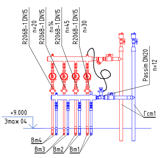
Настройки регулирующей арматуры УУ1.4
