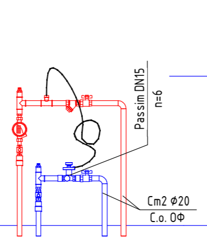
Настройки регулирующей арматуры УЧ ОФ2
