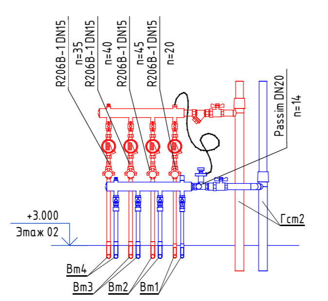
Настройки регулирующей арматуры УЧ2.2
