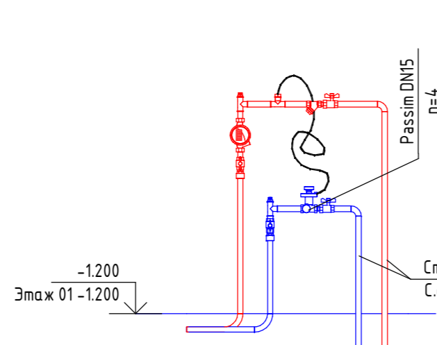
Настройки регулирующей арматуры УЧ ОФ1
