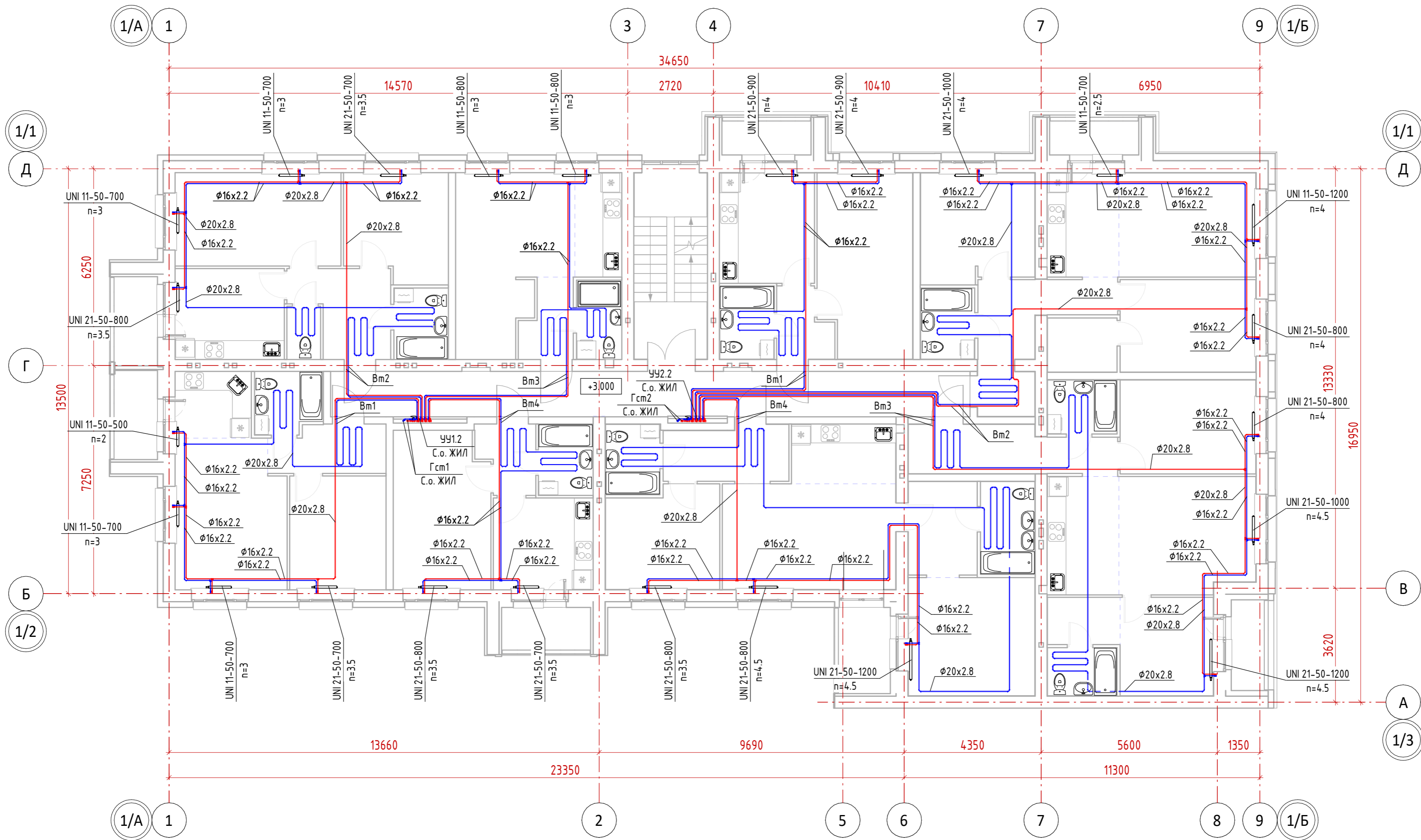
Настройки регулирующей арматуры УЧ1.2
