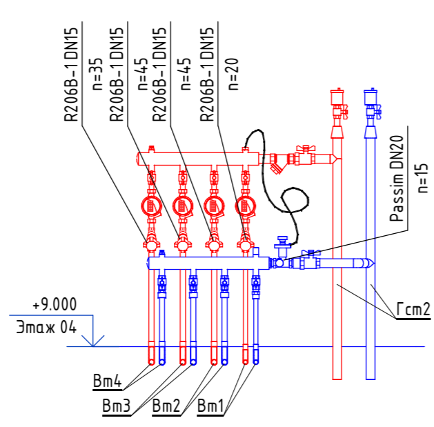
Настройки регулирующей арматуры УУ2.4
