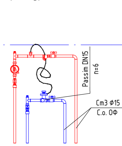
Настройки регулирующей арматуры УЧ ОФ3
