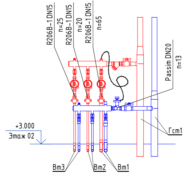
Настройки регулирующей арматуры УЧ1.2
