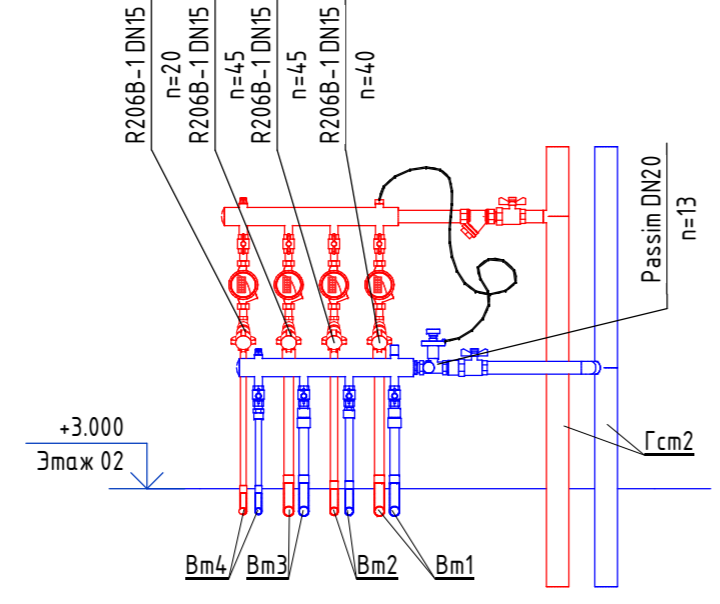
Настройки регулирующей арматуры УЧ2.2
