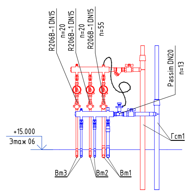
Настройки регулирующей арматуры ЧУ1.6
