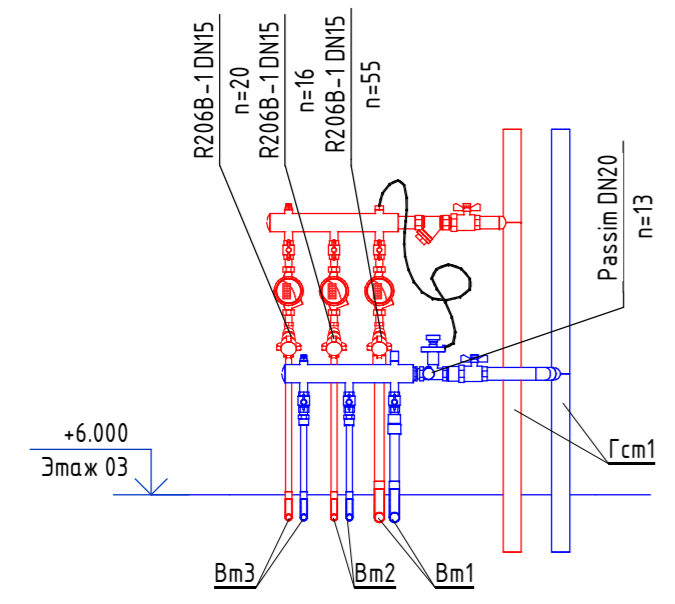
Настройки регулирующей арматуры УЧ1.3
