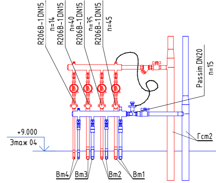
Настройки регулирующей арматуры УЧ2.4
