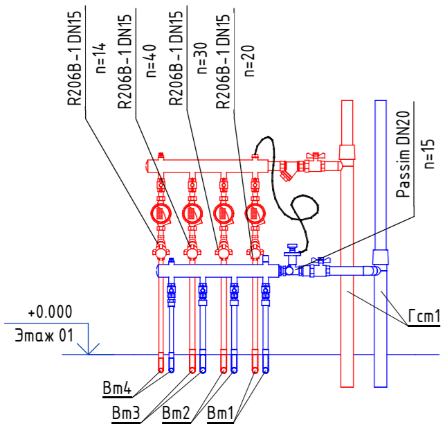
Настройки регулирующей арматуры УЧ1.1
