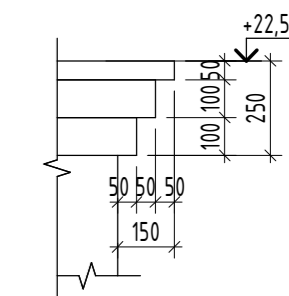
Профиль П5 ( 1 : 20)
