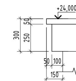
Профиль П5 ( 1 : 20)
