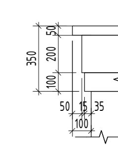
Профиль П6 ( 1 : 20)
