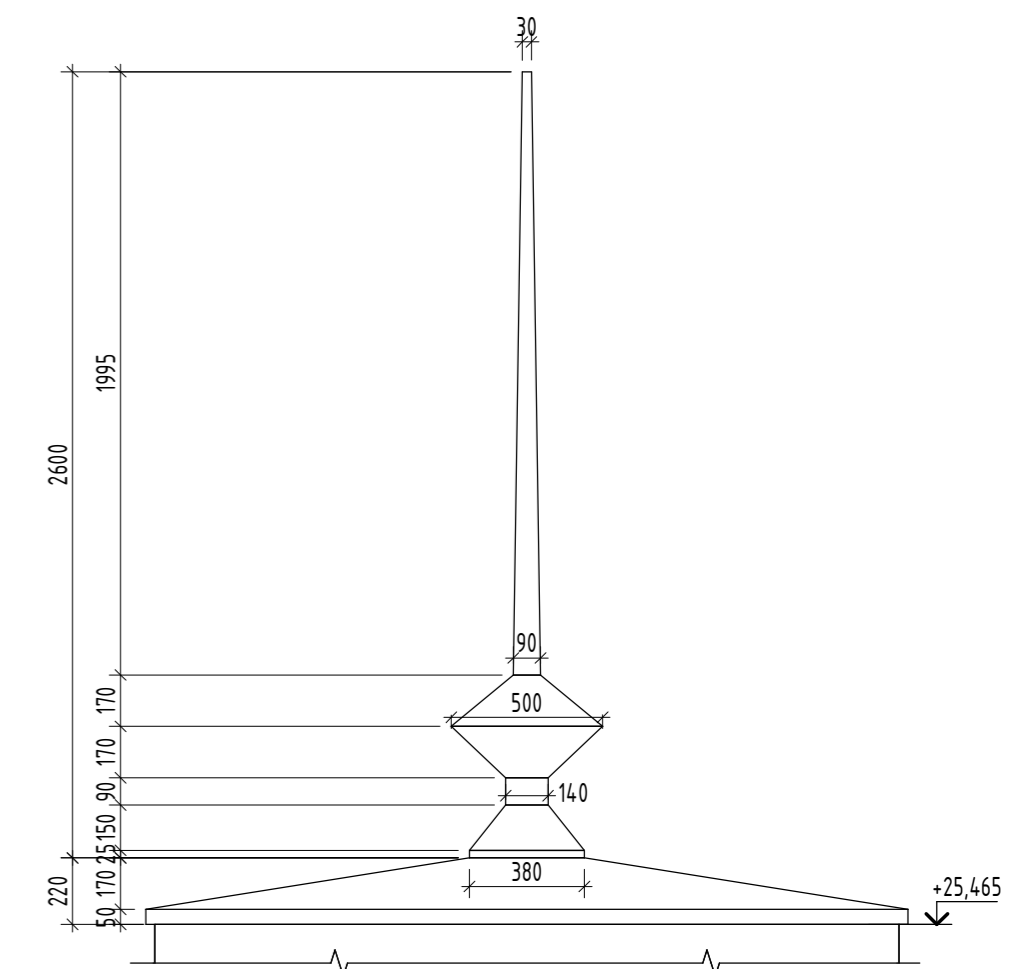
Шпиль (1:25)
