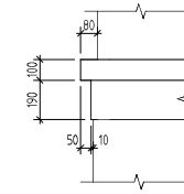
Карниз К4 (1 : 20)
