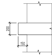
Карниз К6 (1 : 20)
