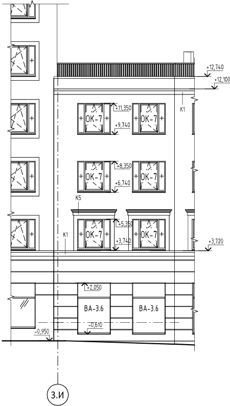
Маркировочный Фасад 3.И-3.Е (Секция 3)
